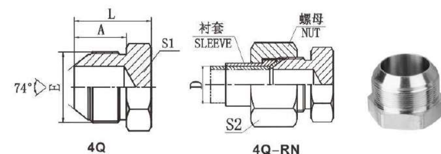
公制外螺纹74° 外锥堵头 METRIC MALE 74° CONE PLUG
