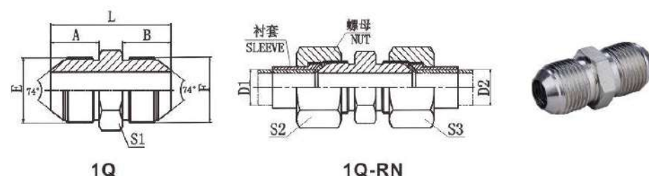
公制外螺纹74° 外锥 METRIC MALE 74° CONE
