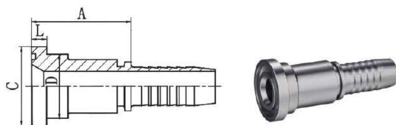
87311 SAE 法兰 3000 PSI SAE FLANGE 3000 PSI ISO12151-3-SAE J516
