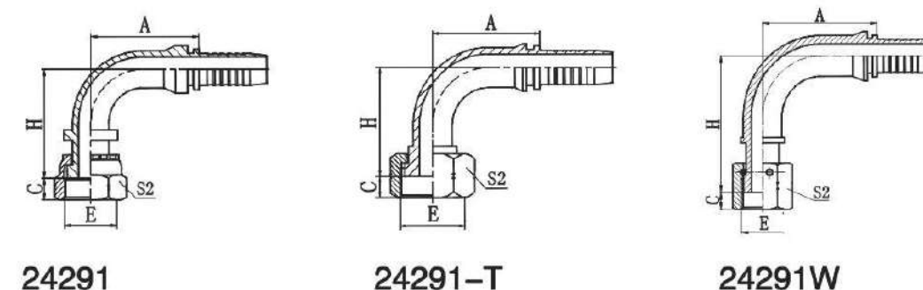
90° 美制ORFS内螺纹平面 90° ORFS FEMALE FLAT SEAT ISO 12151-1—SAE J516
