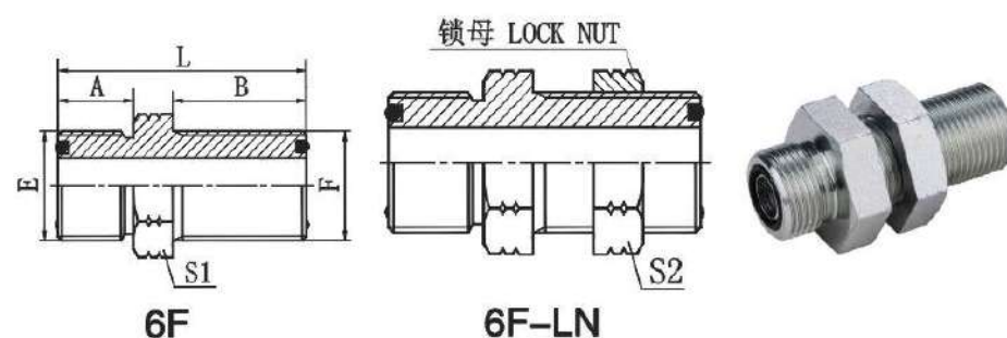
美制ORFS外螺纹 O形圈平面密封过板接头 ORFS MALE O-RING BULKHEAD
