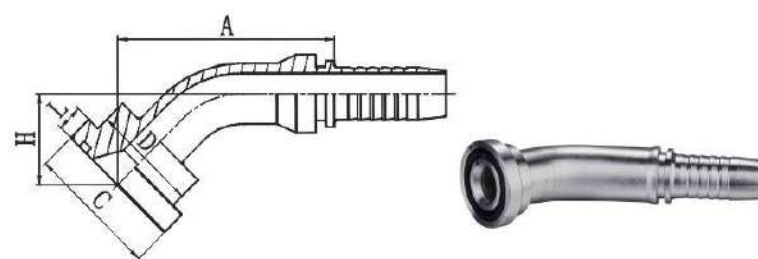
87341 45° SAE 法兰3000 PSI 45° SAE FLANGE 3000 PSI ISO12151-3-SAE J516
