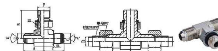
AJOJ-OG 美制JIC外螺纹74° 外锥/ SAE外螺纹带O形圈 轻系列ISO 11926-3分支三通 JIC MALE 74° CONE / SAE O-RING BOSS L-SERIES ISO 11926-3 BRANCH TEE
