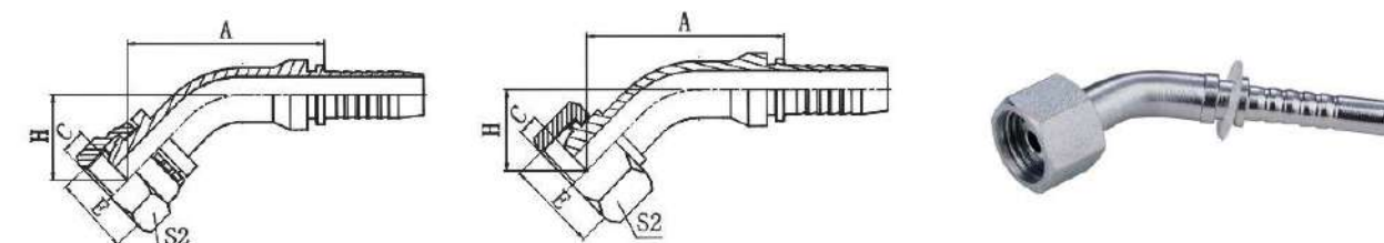
45° 公制内螺纹球面 45° METRIC FEMALE MULTISEAL
