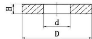
压力表紫铜垫片 Gauge copper gasket
