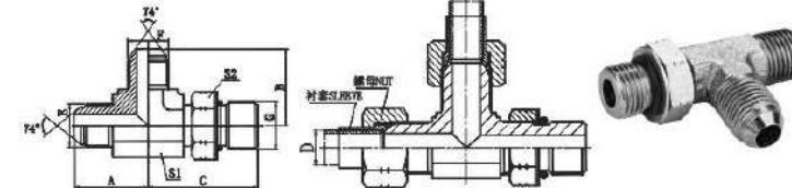
AJJO-OG 美制JIC外螺纹74° 外锥/ SAE外螺纹带O形 圈轻系列ISO 11926-3主支三通 JIC MALE 74° CONE / SAE O-RING BOSS L-SERIES ISO 11926-3 RUN TEE
