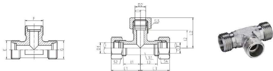
三通接头 EQUAL TEES
