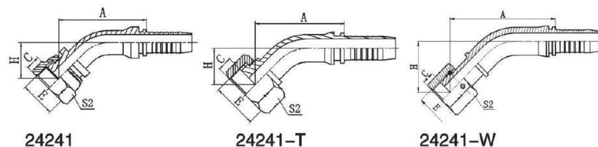
45° 美制ORFS内螺纹平面 45° ORFS FEMALE FLAT SEAT ISO 12151-1—SAE J516
