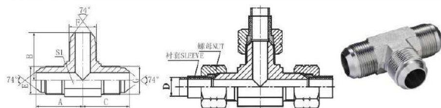
AJ 美制JIC外螺纹74° 外锥三通 JIC MALE 74° CONE TEE
